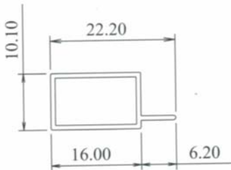
IS155 0.132 kg/m AP : 63 mm
