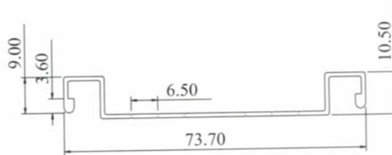
IS412 0.316 kg/m AP : 117 mm
