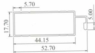
IS413 0.416 kg/m AP : 154 mm
