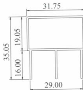
IS6331 0.412 kg/m AP : 195 mm
