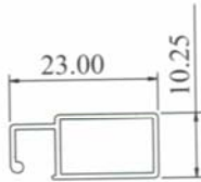
IS1001/SJ156 0.142 kg/m AP : 81.28 mm
