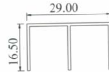
IS1002/Head 0.188 kg/m AP : 153 mm
